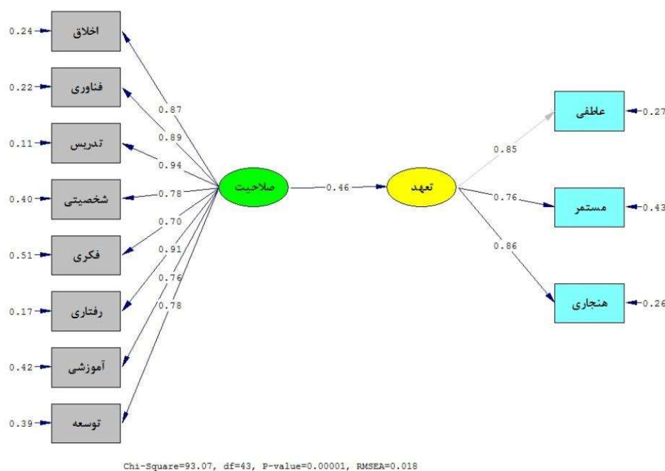
شکل (۱): مدل معادلات ساختاری برحسب ضریب استاندارد
