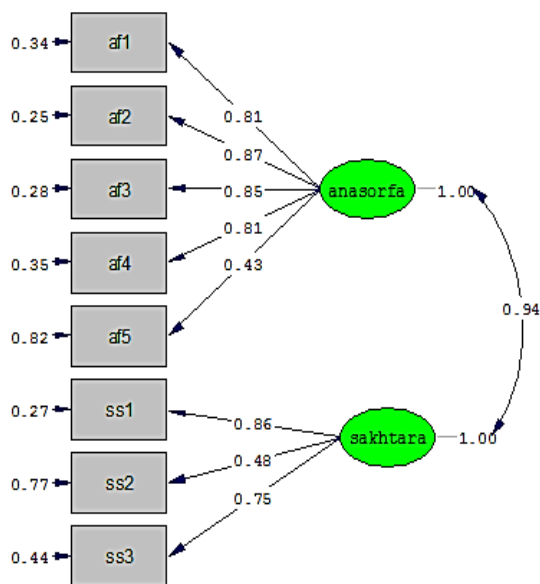
شکل ۲: تحلیل عاملی تاییدی مرتبه اول برای شرایط علی
