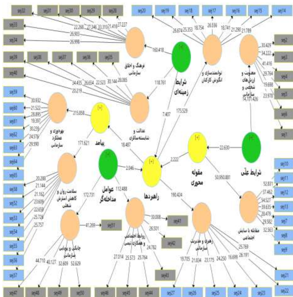
شکل ۳- آماره T مدل کلی پژوهش با تکنیک بوت استرایپینگ
